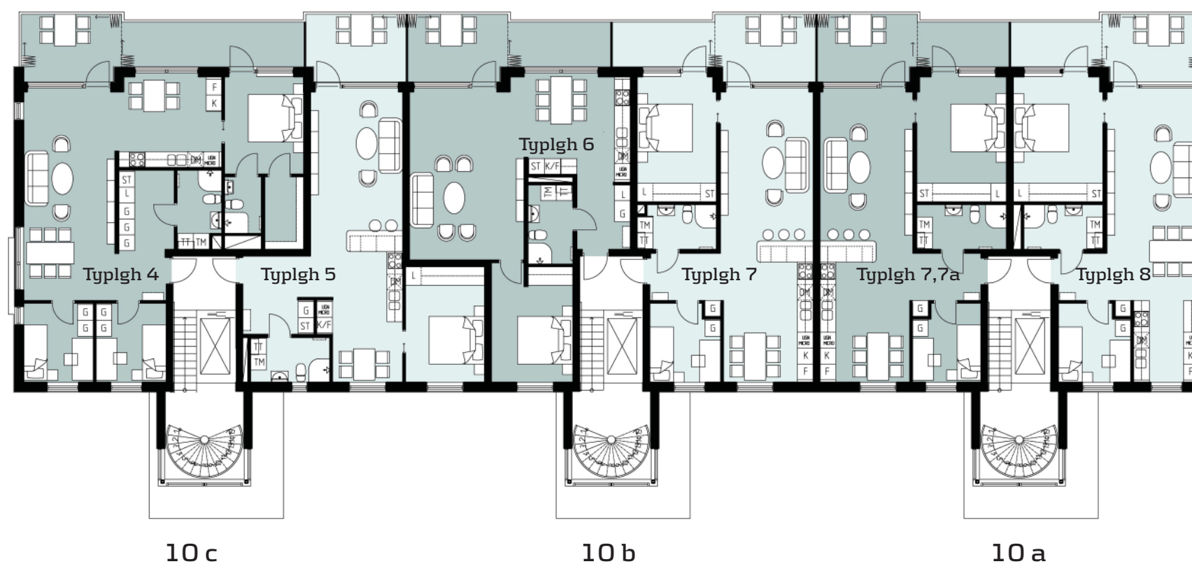
Översikt plan 4-5 Skala 1:200
